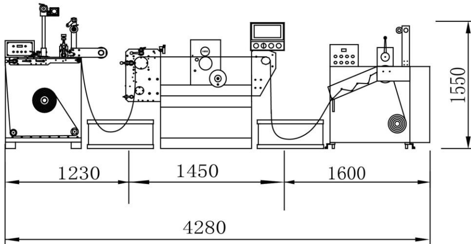
JSL-380间歇式圆模切机示意图
